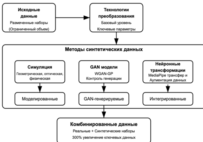
Рис. 12. Создание синтетических жестов с применением генеративных состязательных сетей
